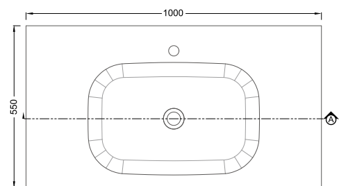
RLHZ1006 SIZE:1000mm×550mm×177mm
