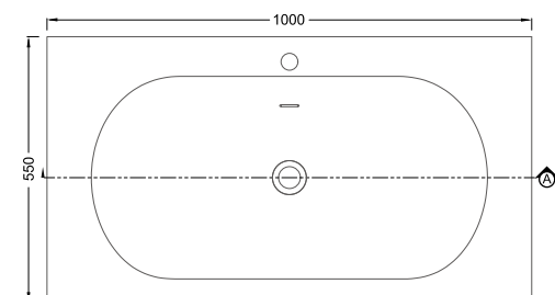
RLHZ1009 SIZE:1000mm×550mm×162mm
