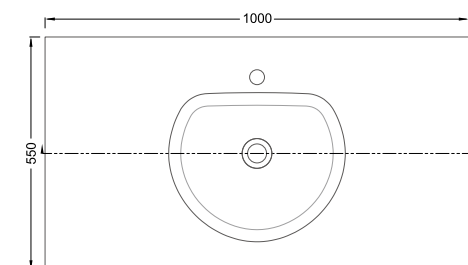
RLHZ1005 SIZE:1000mm×550mm×153mm
