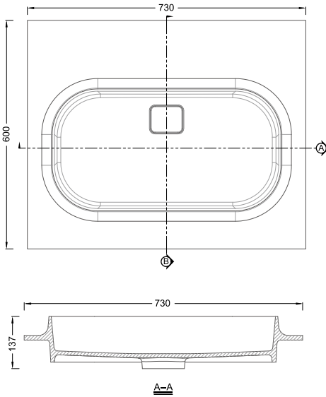
RLC174 SIZE:730mm×600mm×137mm
