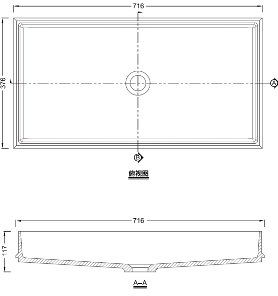
GDRLX003 SIZE:716mm×376mm×117mm
