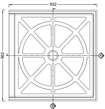
RLF136 SIZE:932mm×962mm×108mm
