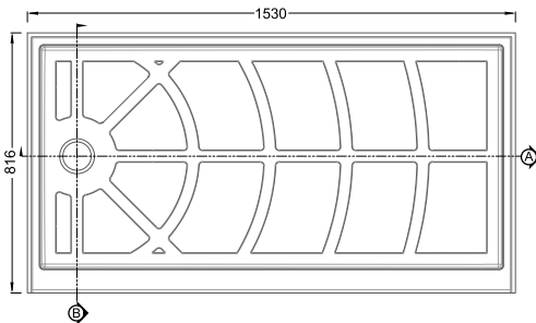
RLF137 SIZE:1530mm×816mm×163mm
