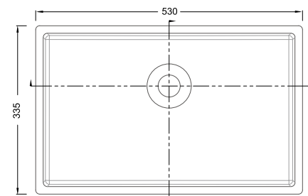
RLB201 SIZE:530mm×335mm×130mm
