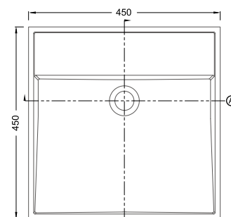
RLB305 SIZE:450mm×450mm×152mm
