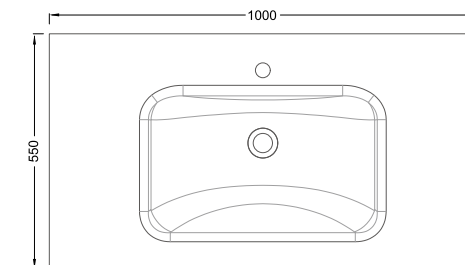
RLHZ1003 SIZE:1000mm×550mm×172mm
