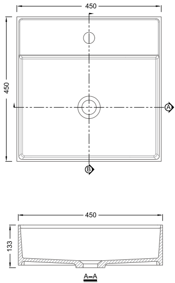
RLC178 SIZE:450mm×450mm×133mm
