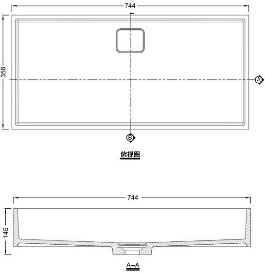
RLB406 SIZE:744mm×358mm×145mm
