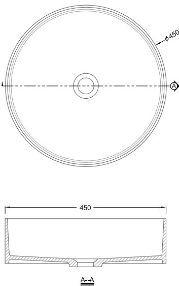
RLA371 SIZE:450mm×450mm×134mm
