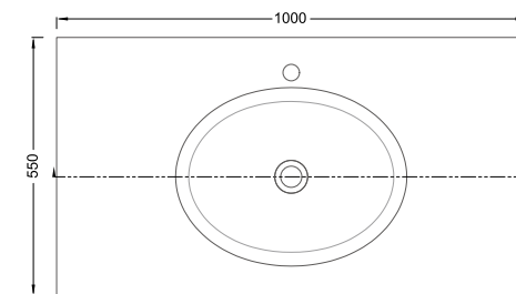
RLHZ1002 SIZE:1000mm×550mm×173mm
