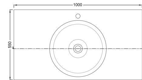
RLHZ1004 SIZE:1000mm×550mm×148mm
