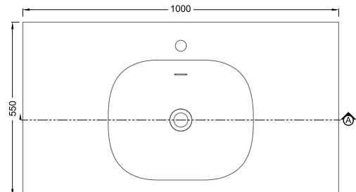
RLHZ1008 SIZE:1000mm×550mm×162mm
